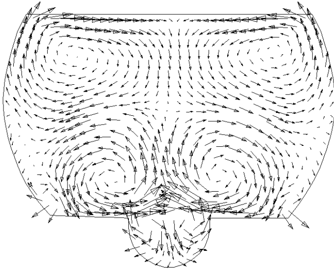
Verteilung der Geschwindigkeiten in einem offenen Gerinnequerschnitt
